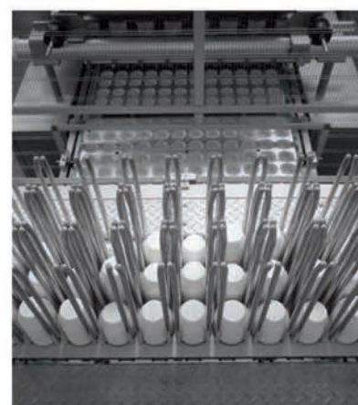
■ Magasin 3 rangées (vue du dessus)
