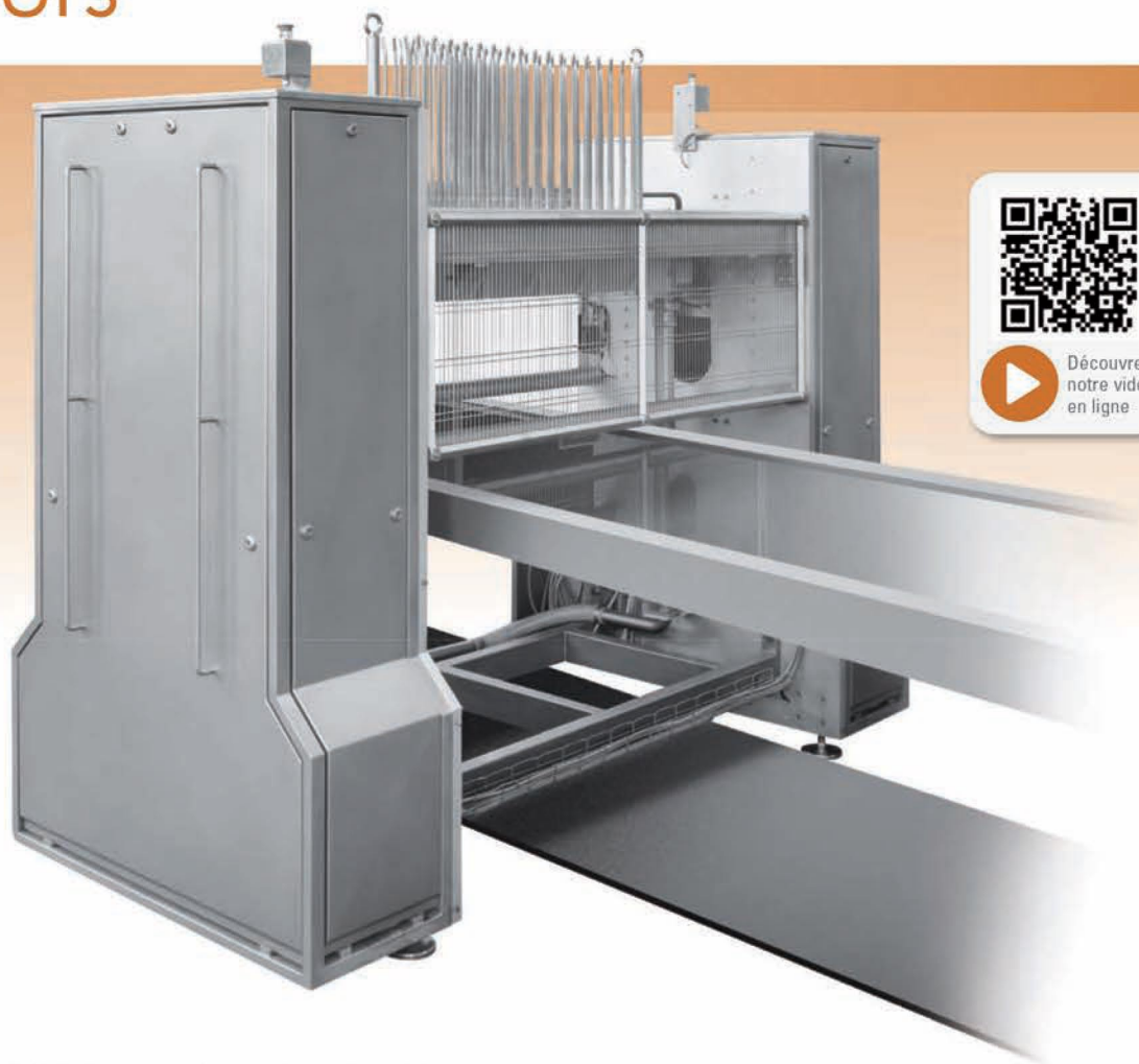
■ Dépilleur moules papier, aluminium
